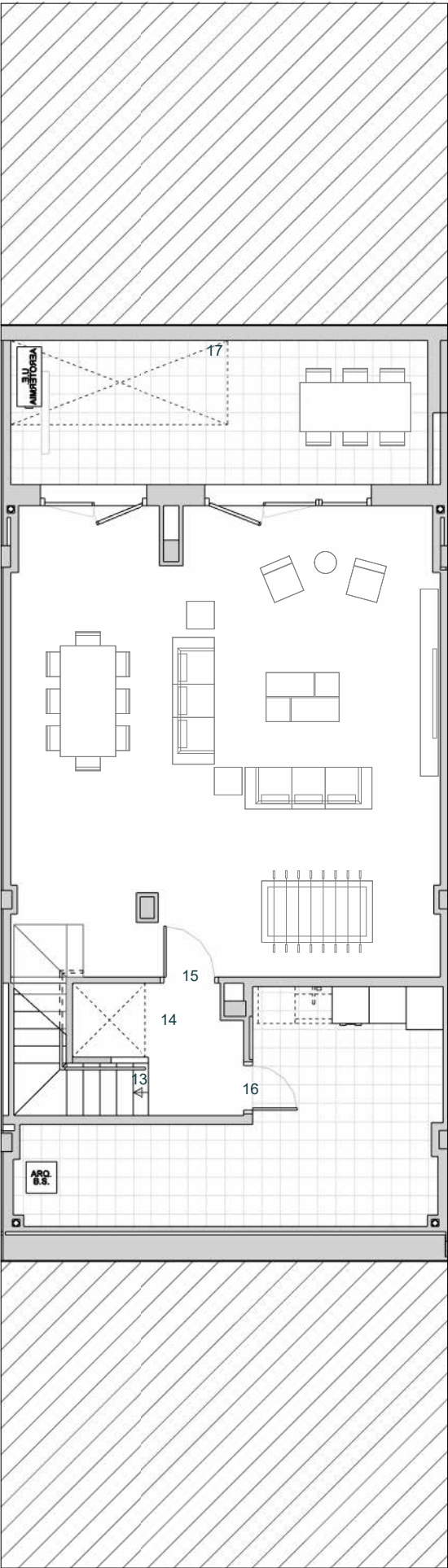
PLANTA SÓTANO
