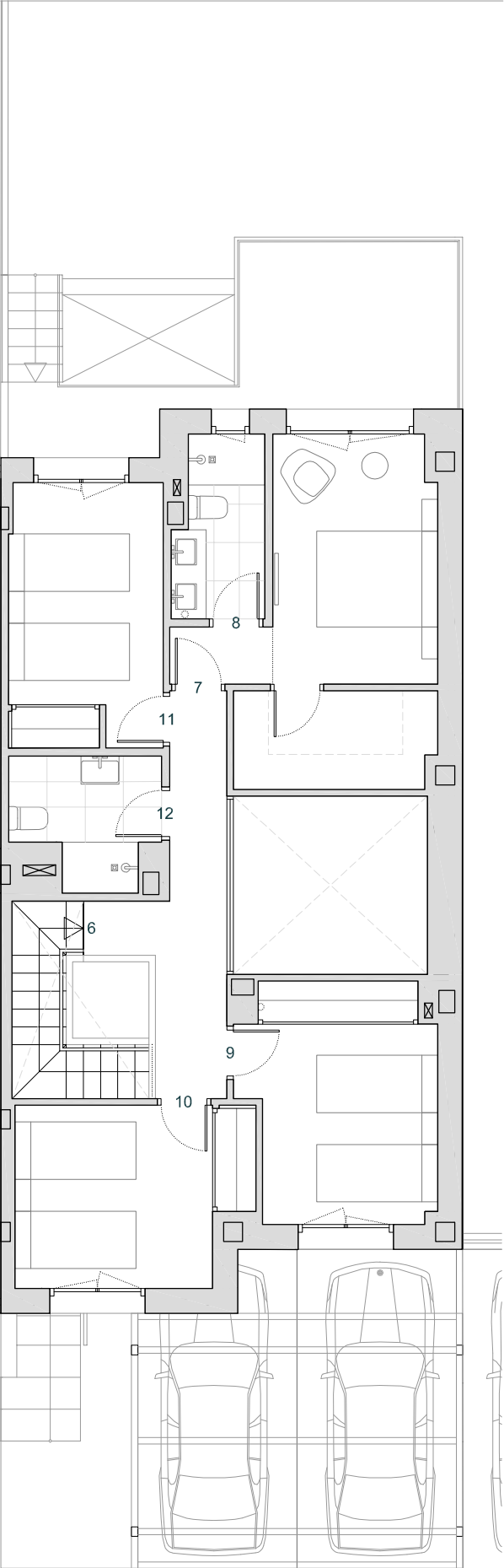
PLANTA PRIMERA
