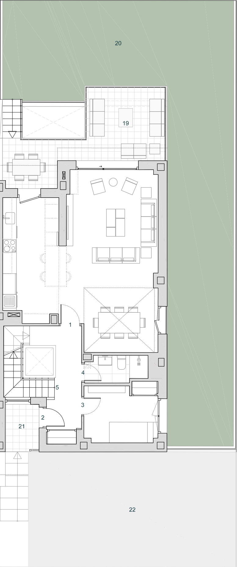
PLANTA BAJA
